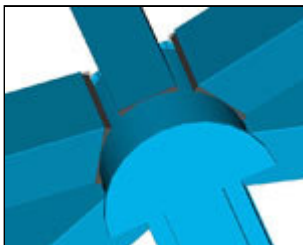
Sposób połączenia 5 krokwi w jednym punkcie (widok z wnętrza ogrodu zimowego)
